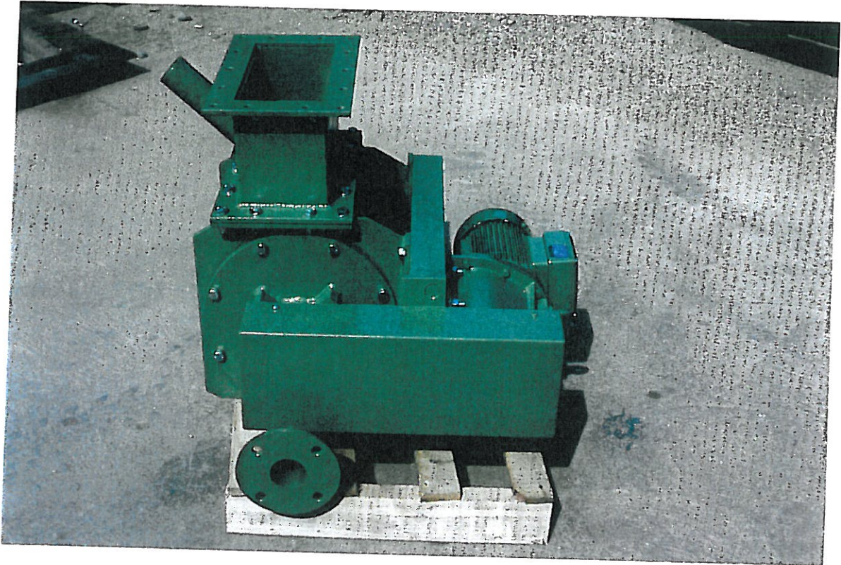
Durchblasseleuse rechteckig, Getriebemotor mit Kettentrieb, Flanschluftsammlkasten, Blasrohr mit Flanschanschluß
