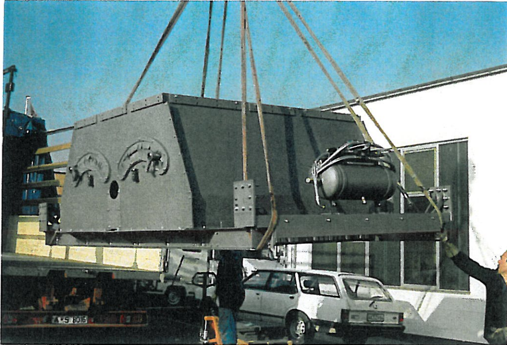
Doppelsegmentverschluß 1800 x 1800 mit Staubschutzkasten
