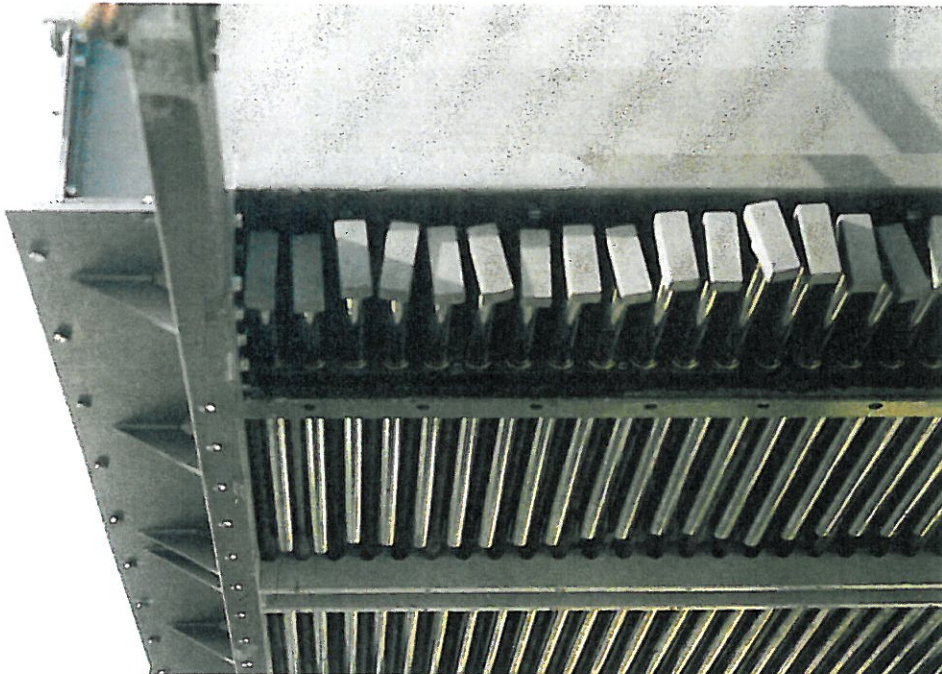
Doppelsegmentverschluß mit darüberliegendem Nadelwehr
